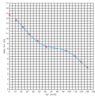
Charakteristika ventilátora
