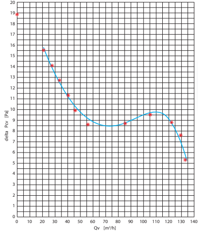
Charakteristika ventilátora
