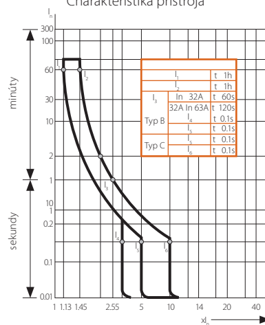
Charakteristika prístroja
