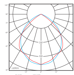
krivky svetivosti \eta = 68\%
