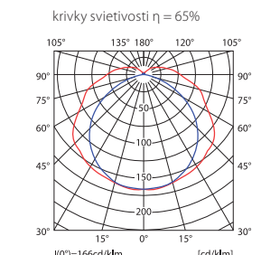
krivky svetivosti η = 65%
