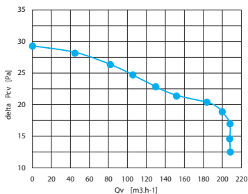
Charakteristika ventilátora
