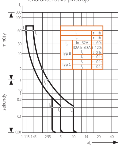
Charakteristika prístroja
