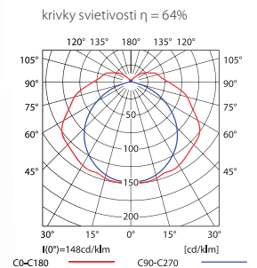
krivky svetivosti η = 64%
