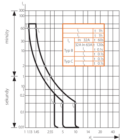
Charakteristika prístroja
