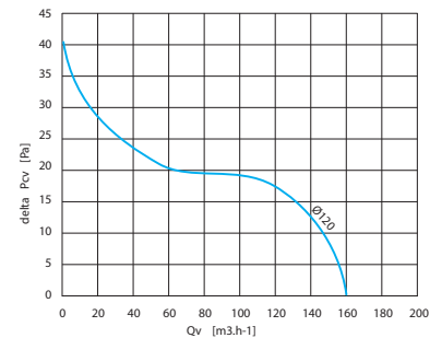
Charakteristika ventilátora
